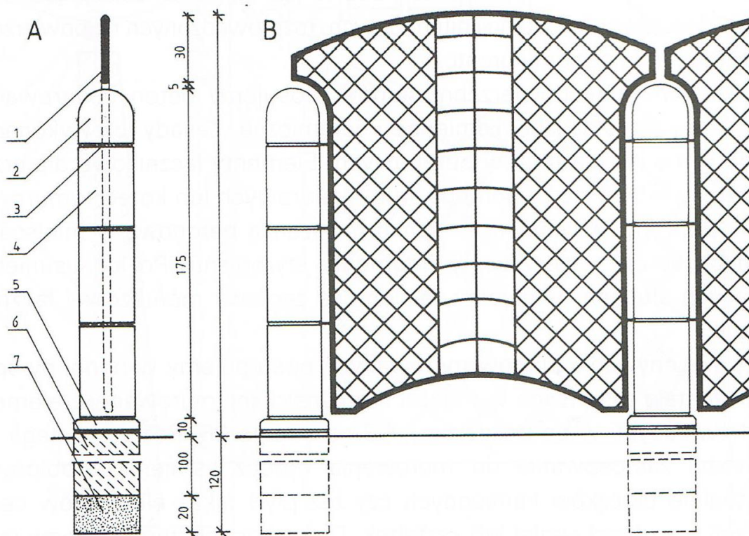
Ryc. 37. Przekrój trejażu o konstrukcji murowanej z elementami metalowymi: A – przekrój; B – widok; 1 – krata stalowa; 2 – kamienny element wieńczący; 3 – zaprawa cementowa; 4 – blok kamienny; 5 – kamienna podstawa słupa; 6 – fundament betonowy; 7 – piasek (K. G.)
