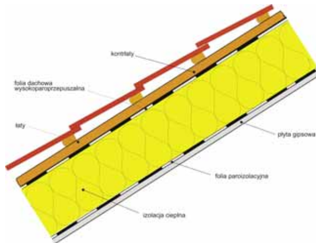
Typowy układ warstwy połaci dachu, bez poszycia
