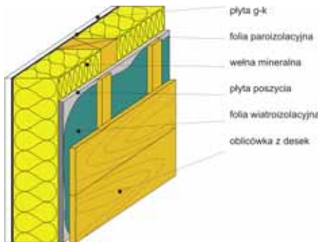
Układ warstw ściany z okładziną drewnianą
