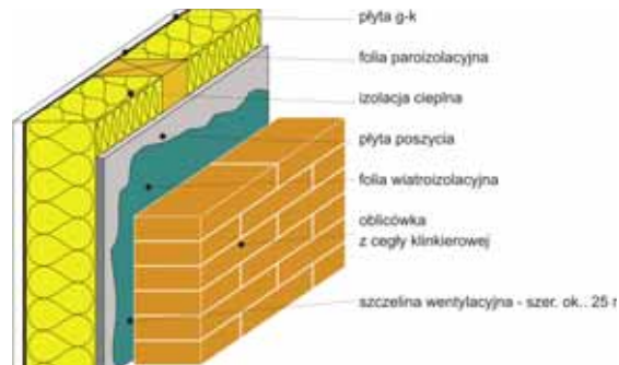
Układ warstw ściany z okładziną ceglana
