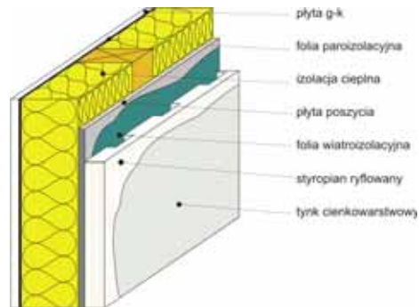
Układ warstw ściany z okładziną styropianową i tynkiem
