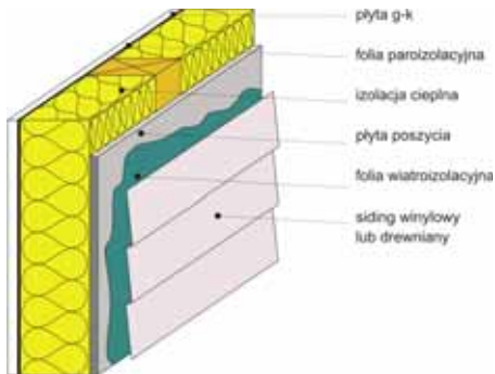
Układ warstw ściany z okładziną winylową
