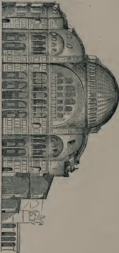
91 Kościół św. Zofii. Przekrój.
