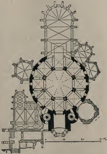
169. Kaplica zamkowa w Akwizgranie. Plan poziomy.
