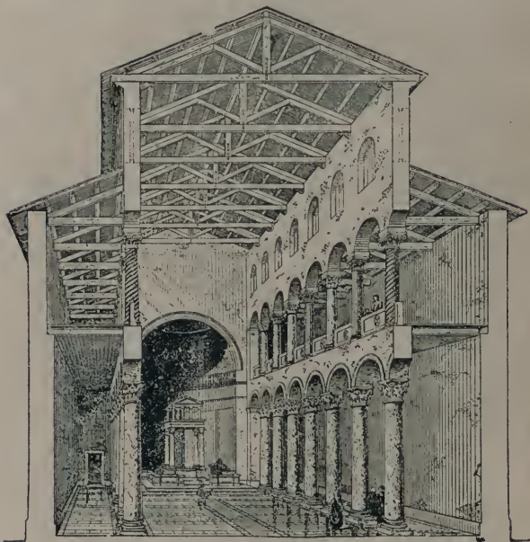
79. Przekrój bazyliki św. Agnieszki w Rzymie.
