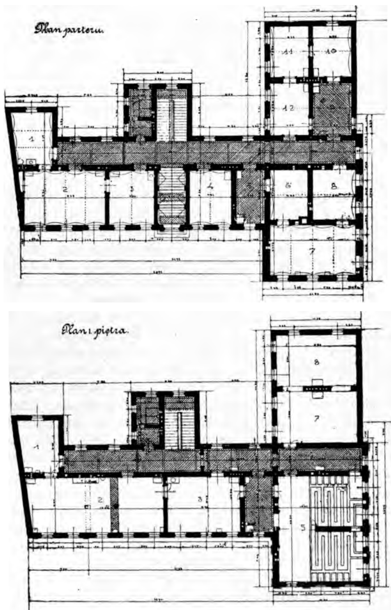
Plany Zakładu.
