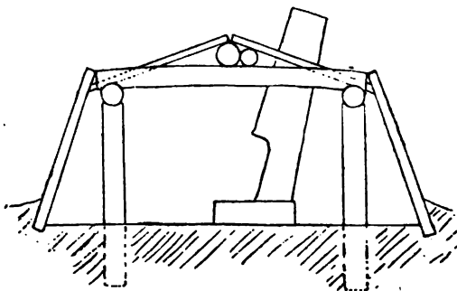
Rys. 66. Szkielec jurty.
