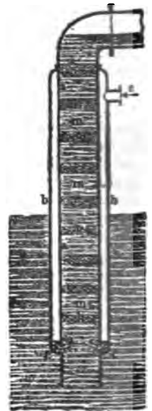
Pompa mamutowa.
