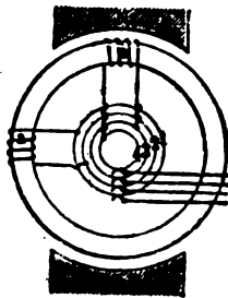
Fig. 10. Schemat maszyny wielofazowej.
