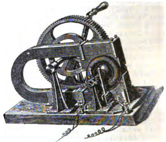
Fig. 4. Machina magneto-elektryczna Gramme'a 1870.
