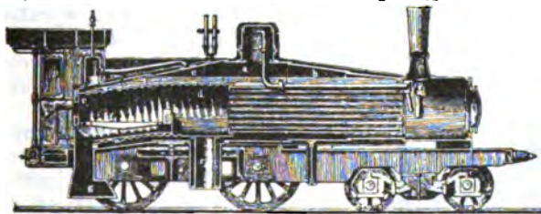
Fig. 4. Lokomotywa Lentza w przecięciu.
