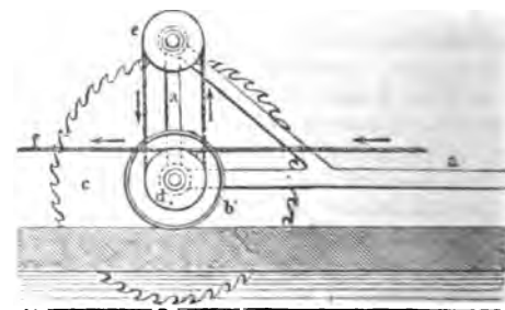
Fig. 2. Pług lodowy, widok z przodu.
