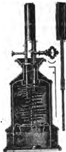
Fig. 2. Lampa z moderatozem.
