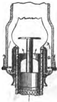
Fig. 7. Lampa Cautiusa.
