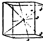
Fig. 9. Romboedr.
