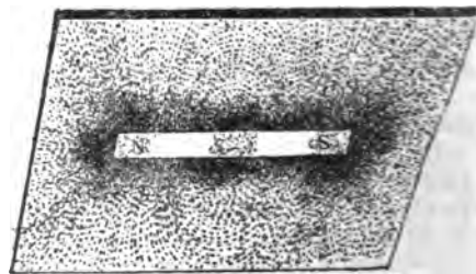
Fig. 3. Linje magnetyczne
