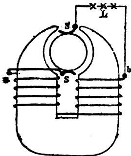
Fig. 5. Pierwszy schemat maszyny dynamo-elektrycznej.
