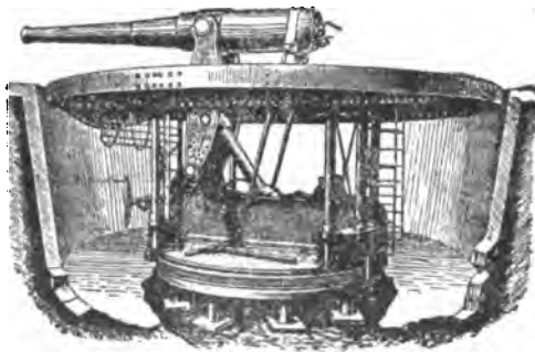
Fig. 6. Laweta hydropneumatyczna.
