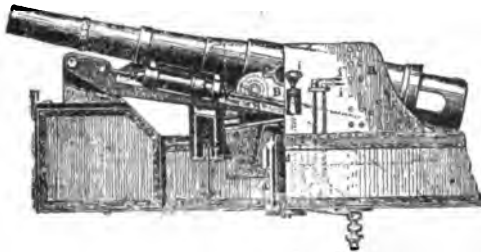
Fig. 5. Laweta hydrauliczna.
