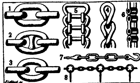
Różne formy łańcuchów.
