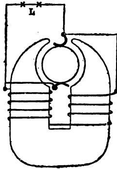
Fig. 6. Drugi schemat maszyny dynamo-elektrycznej.
