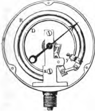
Fig. 3. Manometr rurowo-sprężynowy.
