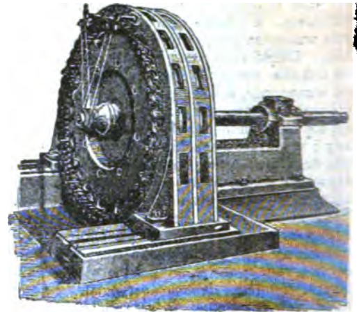
Fig. 11. Machina Oerlikon.
