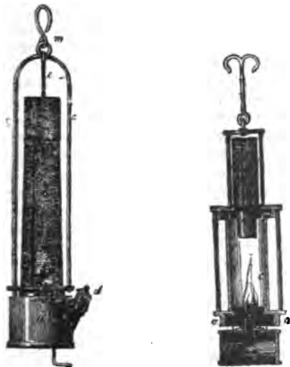
Fig. 1. Lampa Davego. Fig. 2. Lampa Combes'a.
