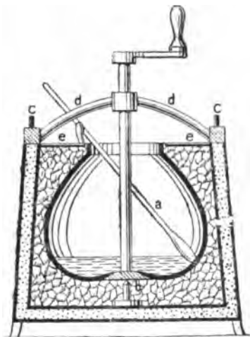
Maszyna do lodów Fullera.
