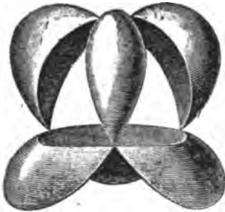
Kummera powierzchnia.
