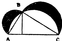
Księżyc Hipokratesa.
