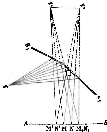
Fig. 2. Doświadczenie Fresnel'a.
