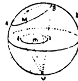
Fig. 1. Rzut stereograficzny.
