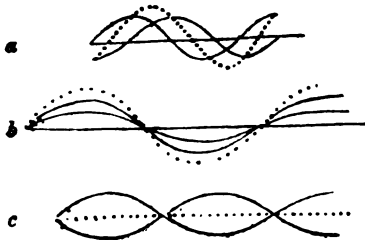
Fig. 1. Krzyżowanie fal.
