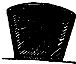
Fig. 1. Kryształizacja siarki przez stopienie.
