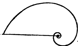
Spiralna logarytmiczna.
