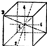
Fig. 5. Sześcian.
