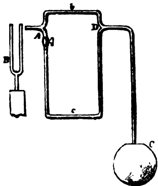
Fig. 3. Przyrząd Kanego do interferencji głosu.
