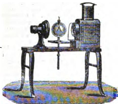
Fig. 2. Sciophtikon.
