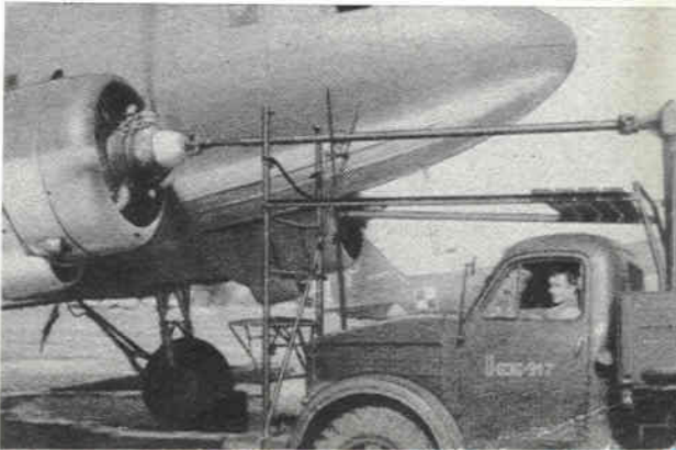
Rozruch silnika przy użyciu samochodu z przystawką (fot. R. Marcinkiewicz)
