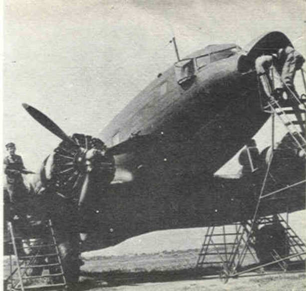
Samolot fotogrametryczny, widoczne wypukłe okno nawigatora, zawierające przyrządy celownicze (fot. WAF - S. Syndoman)
