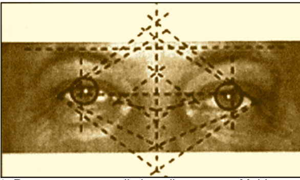
Rys. 11: Parametry geometrii oka odkryte przez Muldaszewa w wokółocnych fragmentach twarzy opierają się na - jednakowej u wszystkich ludzi - wielkości rogówki
