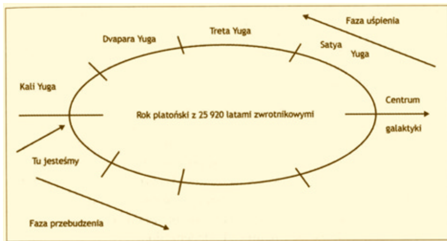
Rys. 86: Układ Słoneczny porusza się ruchem eliptycznym w kierunku centrum galaktyki i ponownie się od niego oddala.
