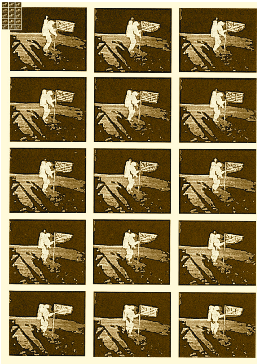
Rys. 1: Choć NASA twierdzi, że Księżyc nie posiada atmosfery, flaga powiewa na wietrze. Dlaczego NASA kłamie? Czy informacje dotyczące Księżyca są niezgodne z prawdą? A może Amerykanie nigdy tam nie byli - tylko w studio?
