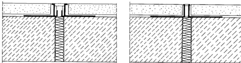
Rys. 12. Profile do dylatacji warstw wierzchnich układanych na cienkiej warstwie zaprawy: a) z wymienną kształtką elastyczną, b) ze stałą wkładką elastyczną [5, s. 433]
