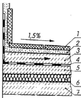
Rys. 5. Przykład podłogi wodoszczelnej na stropie – z instalacją odwadniającą [16, s. 41] 1 – płytki ceramiczne, 2 – zaprawa cementowa, 3 – podkład betonowy, 4 – izolacja wodoszczelna, 5 – warstwa podkładu tworząca spadek, 6 – izolacja cieplna, 7 – strop
