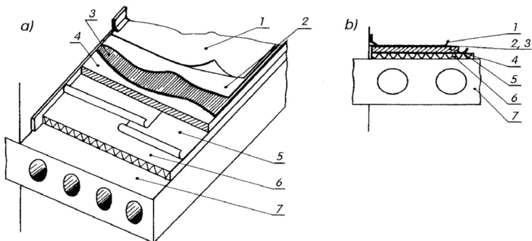
Rys. 21. Podłoga o konstrukcji pływającej z posadzką z wykładziny PVC: a) układ warstw, b) przekrój [16, s. 191] 1 – elastyczna wykładzina PVC, 2 – warstwa kleju, 3 – warstwa szpachłówki wygładzającej podkład, 4 – podkład, 5 – warstwa ochronna, 6 – izolacja przeciwdźwiękowa (wraz z paskiem izolacji wzdłuż ściany)
