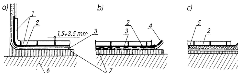
Rys. 7. Podłoga kwasoodporna z posadzką z płytek ceramicznych układanych na kicie asfaltowym: a) podkład gruntowany roztworem asfaltowym, b) izolacja z papy, c) z asfaltu lanego [16, s. 274] 1 – płytki ceramiczne, 2 – kit asfaltowy, 3 – grunt asfaltowy, 4 – papa asfaltowa lub folia, 5 – asfalt lany, 6 – strop, 7 – gładź cementowa
