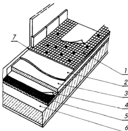
Rys. 23. Podłoga z nawierzchnią z ceramicznych płytek mozaikowych na podkładzie pływającym [16, s. 236] 1 – płytki mozaikowe, 2 – warstwa zaprawy, 3 – podkład cementowy, 4 – papa asfaltowa, 5 – izolacja przeciwdźwiękowa, 6 – strop, 7 – kit elastyczny
