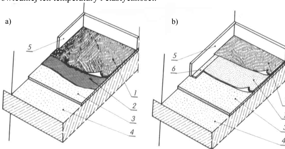
Rys. 22. Posadzki z wykładziny dywanowej: a) przyklejana, b) napinana [16, s. 206] 1 – wykładzina dywanowa, 2 – klej, 3 – podkład, 4 – strop, 5 – listwa cokołowa, 6 – listwa mocująca, 7 – podkładka filcowa
