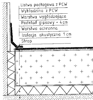
Rys. 3. Podłoga pływająca – na podkładzie z gipsu [6, s. 20]
