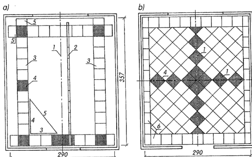
Rys. 14. Rozplanowywanie płytek: a) w układzie prostym, b) w układzie skośnym [16, s. 227]
