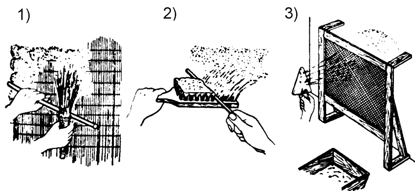
Rys. 9. Wykonywanie tynku nakrapianego: 1) z miotłki, 2) ze szczotki, 3). z kielni przez siatkę [15, s. 329]
