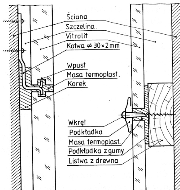
Rys. 12. Mocowanie okładzin szklanych [8, s. 15]
